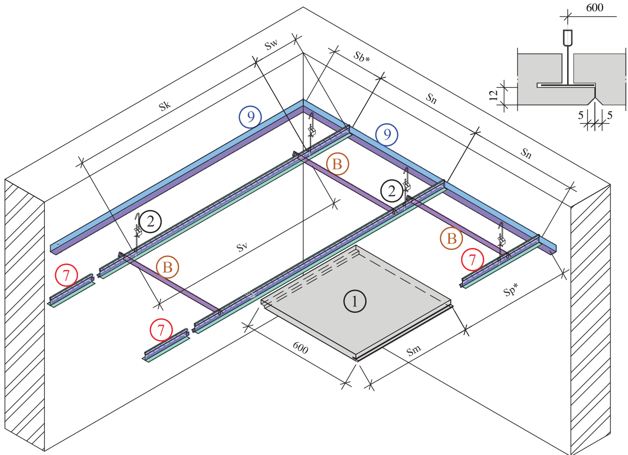
ZFig. 7.2. T-profile frame.
